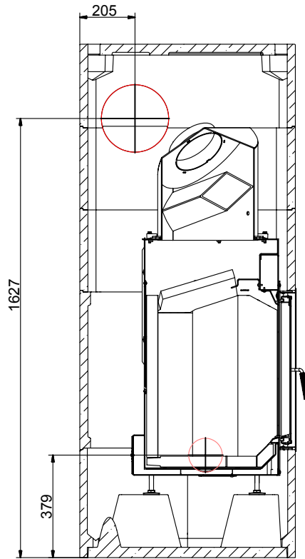
SCHNITT A-A
