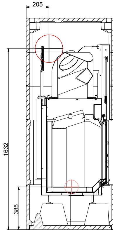
SCHNITT A-A
