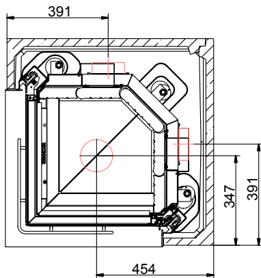
SCHNITT B-B
